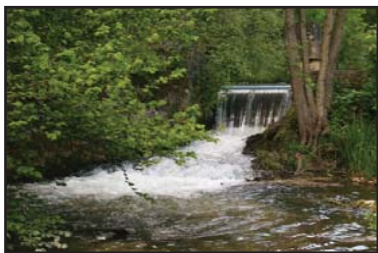
vanne et chute d'eau sur un bief.
